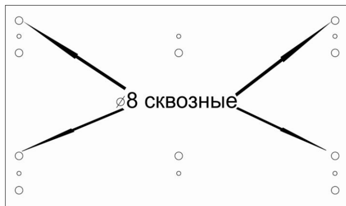
Рис.1 вид снизу
